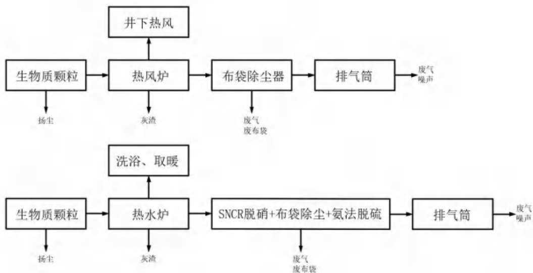
图 2-3 运营期生产工艺流程及产排污节点图
